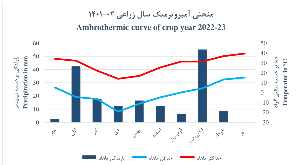
شکل ۱- منحنی آمبروترمیک داده‌های هواشناسی سال زراعی ۱۴۰۱-۰۲ Figure 1. Ambrothermic curve of meteorological data of crop year 2022-23
